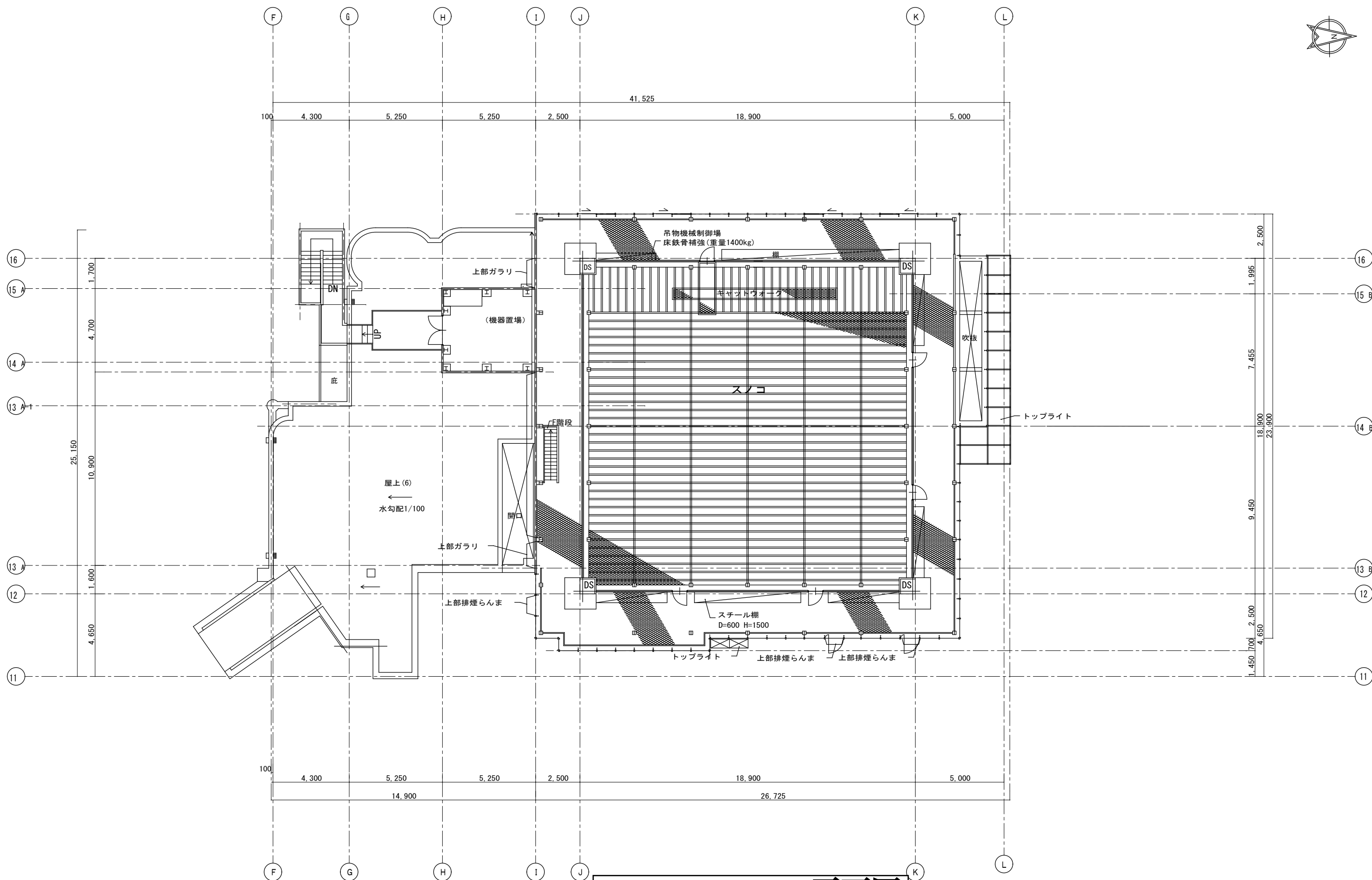
スノコレベル 平面図
