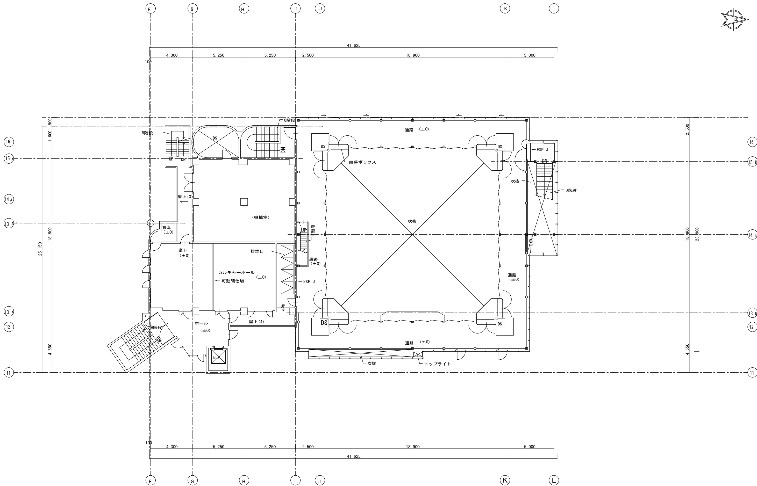
3階 平面図
