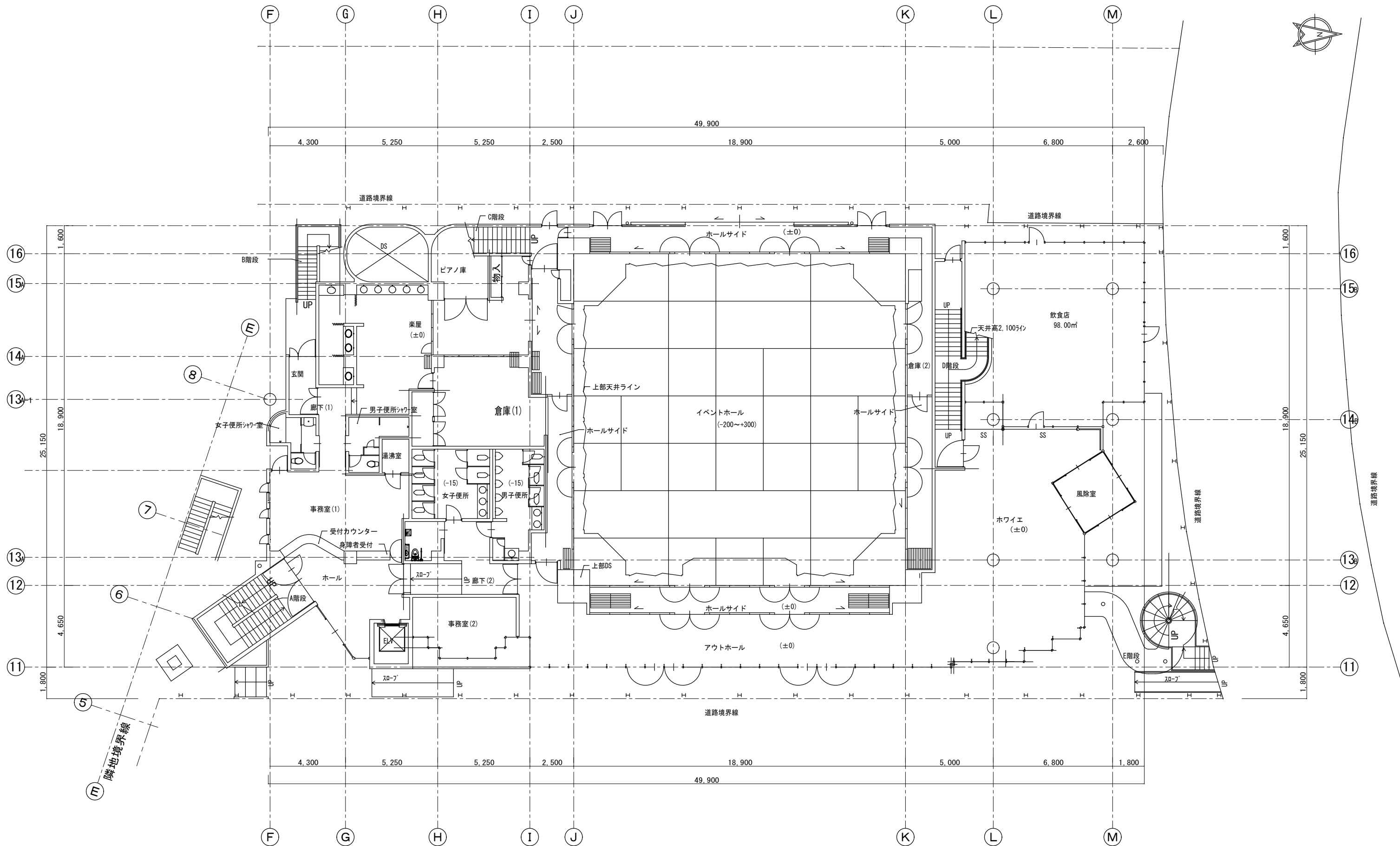
1階 平面図
