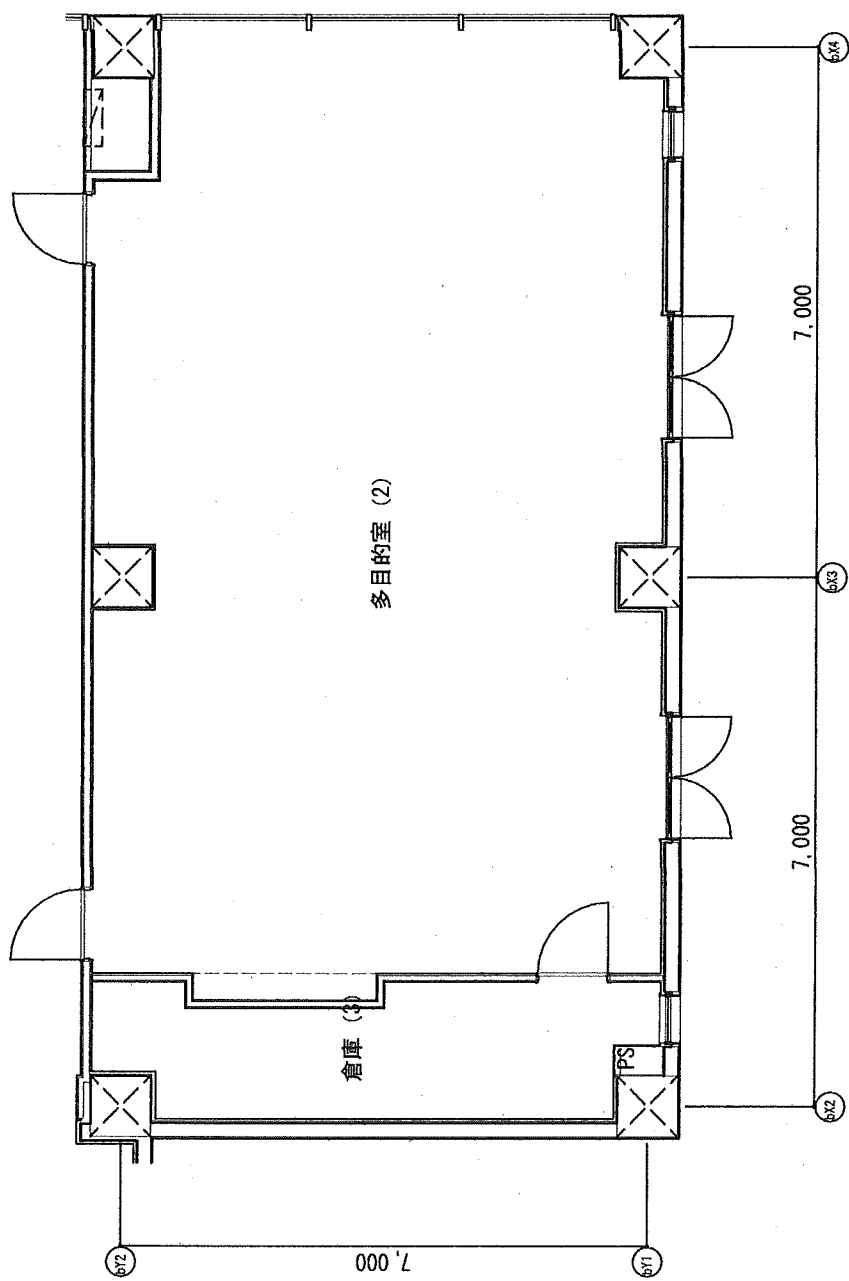
多目的室 1 平面图 1/100
