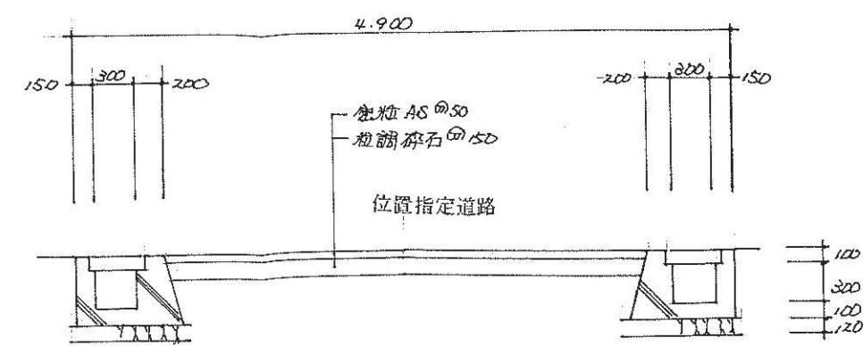
標準断面図 S=1:50
