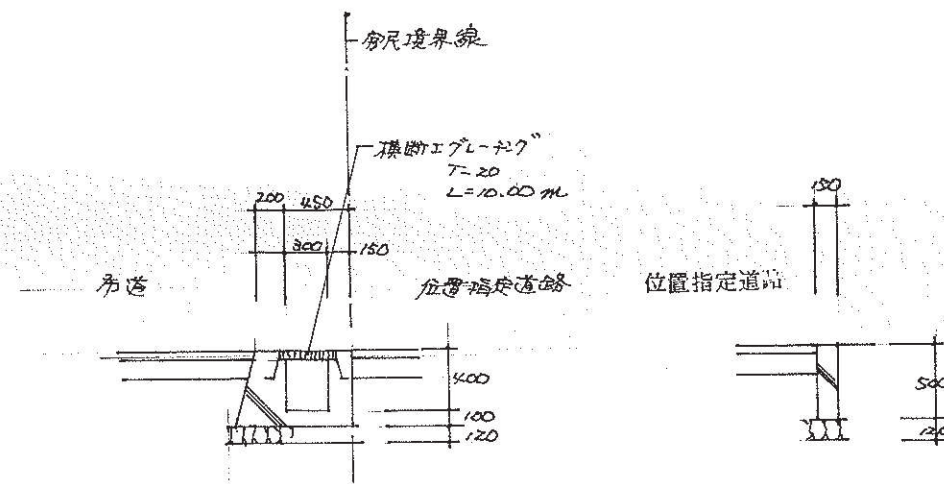
提案断面図 S=1:50
