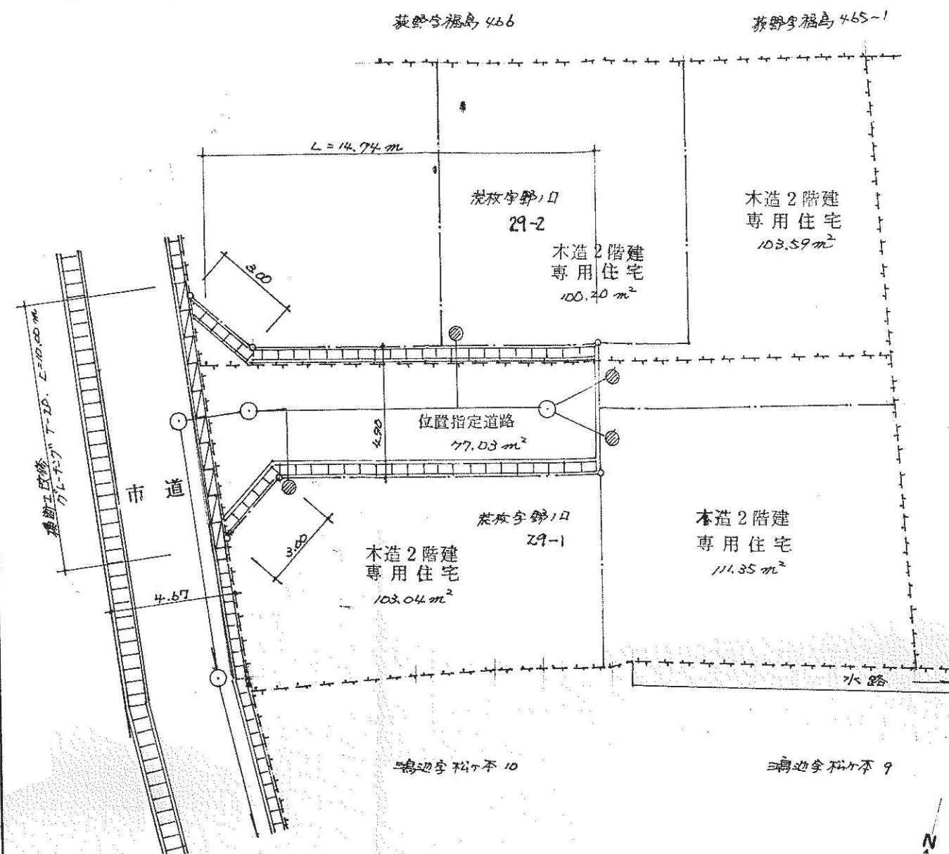
平面図 S=1:200
