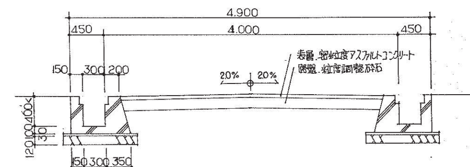
断面図 1:50
