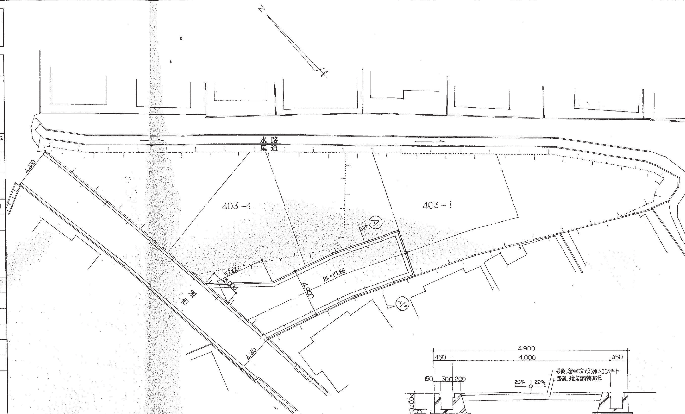
平面図 1:200
