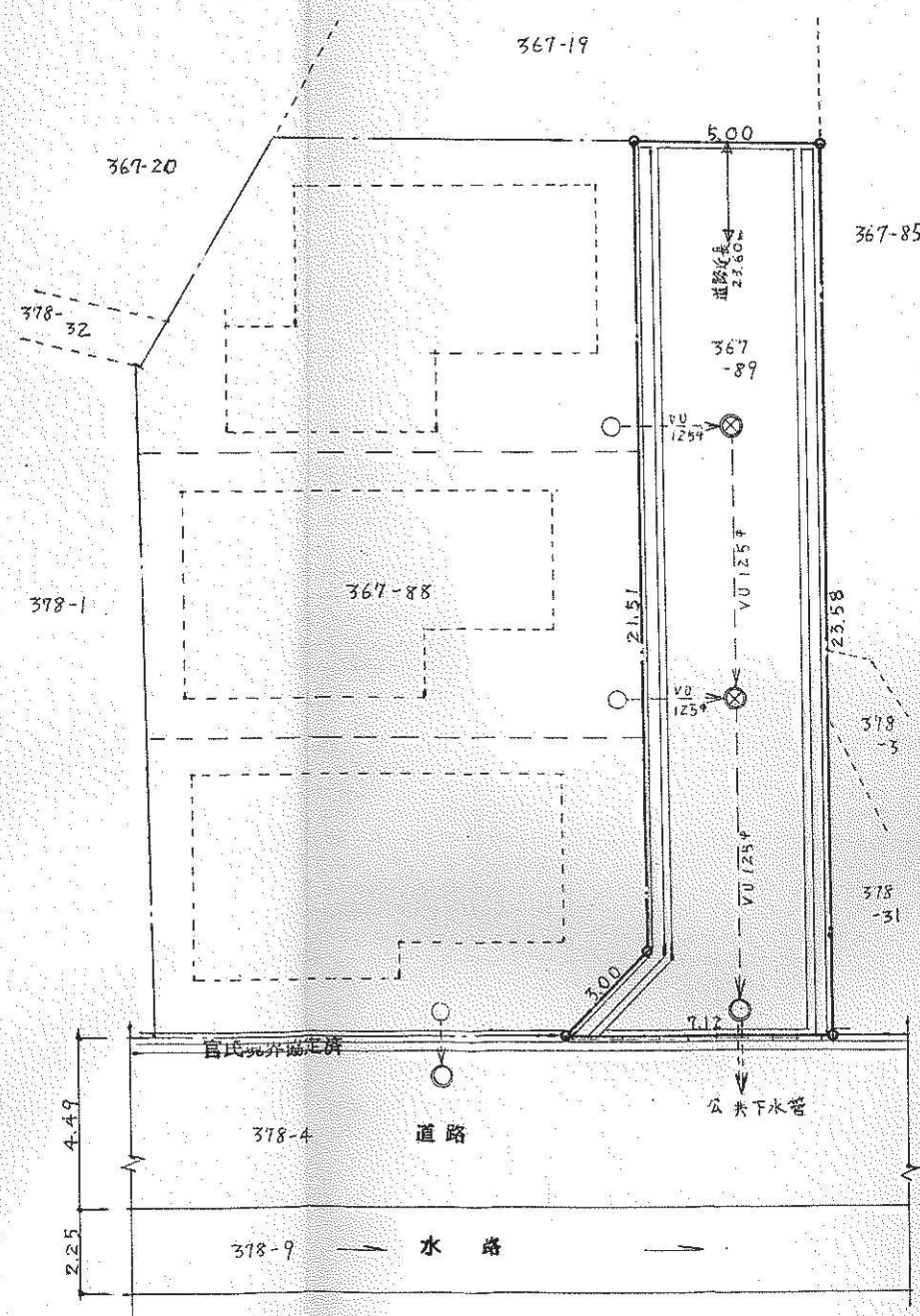
平面図
