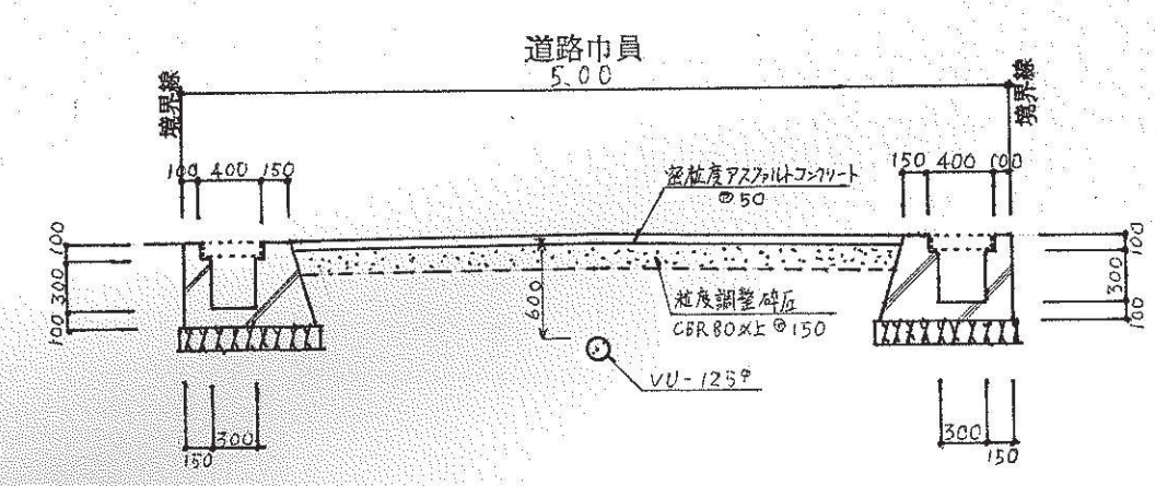
断面図
