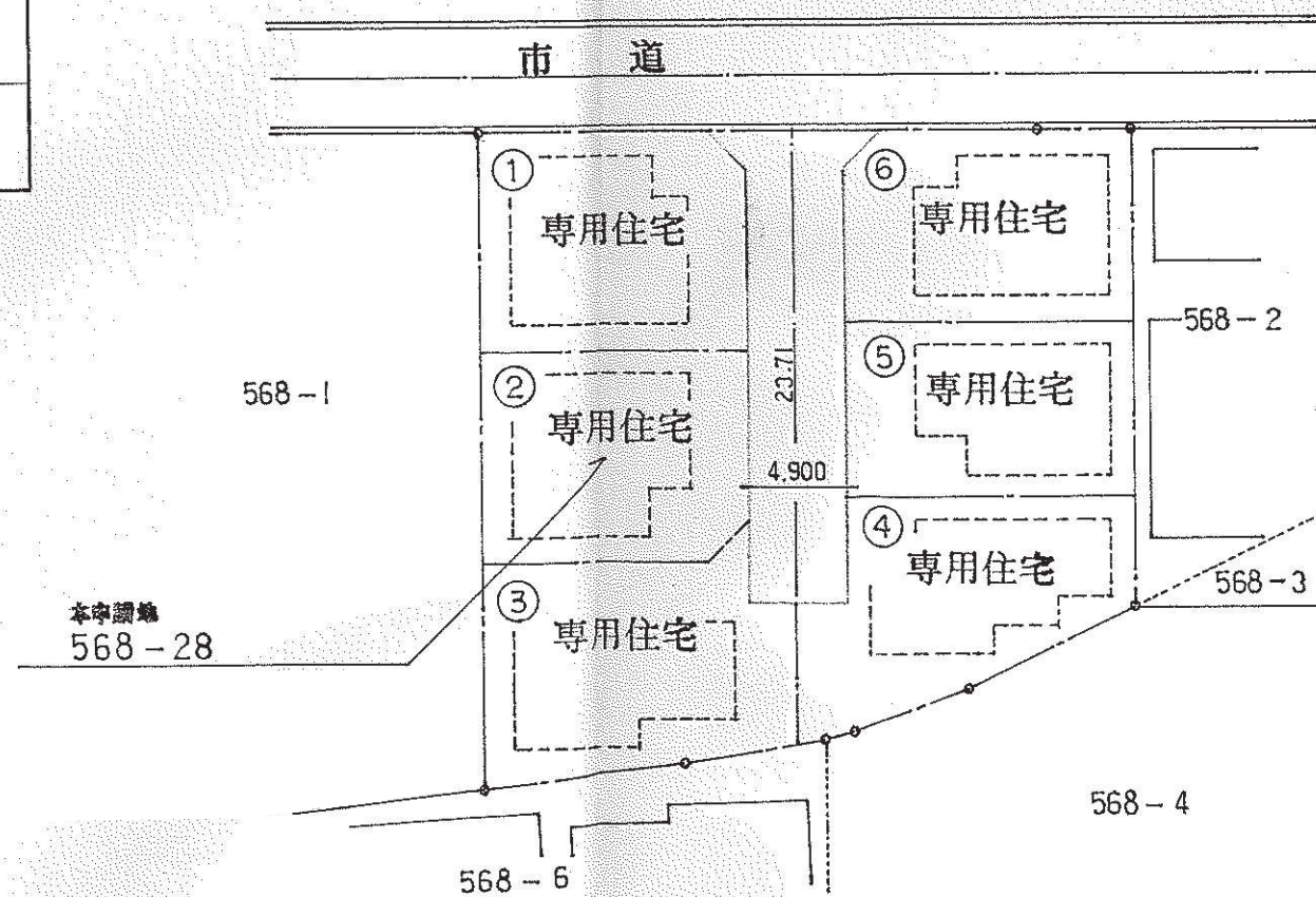
土地利用計画図 1 : 400
