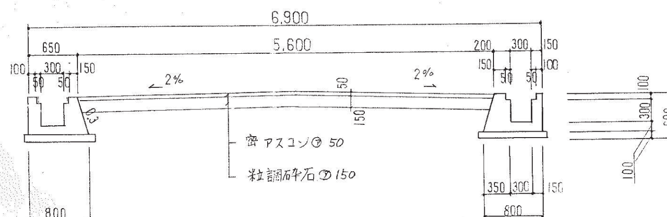
道路横断面 S: 1/50
