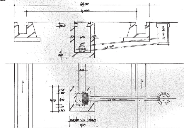
道路構造図 排水施設構造図
