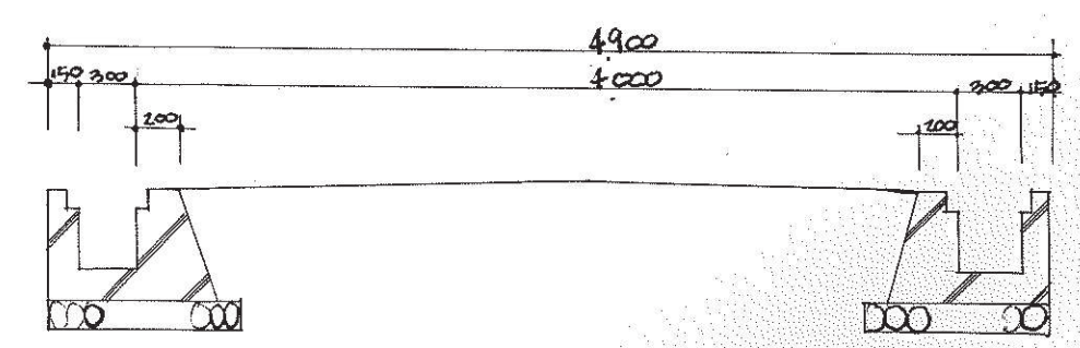
道路標準断面図 S=740
