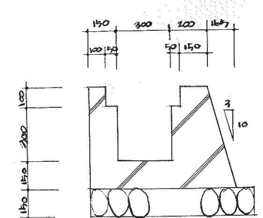
道路標準断面図 S=740
