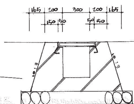
側溝標準断面図 S=740
