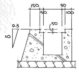
側溝詳細図 S1/30
