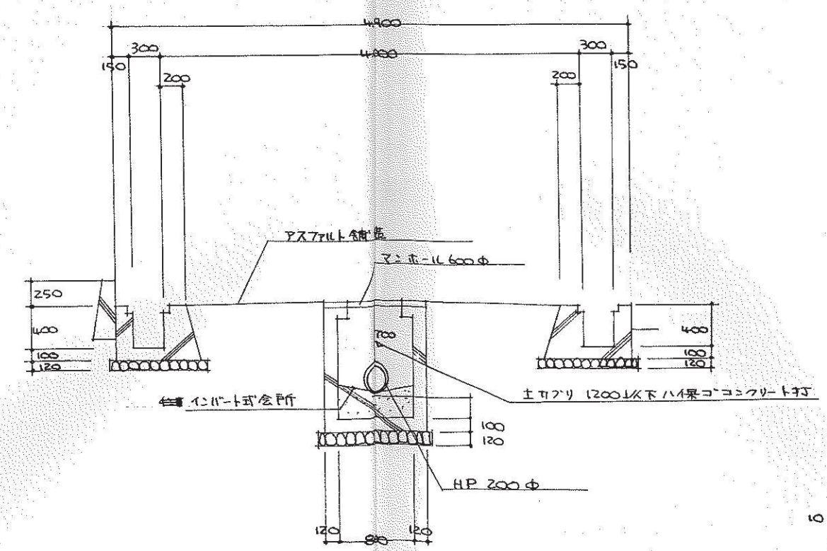
a-a' 道路断面図 S1/50
