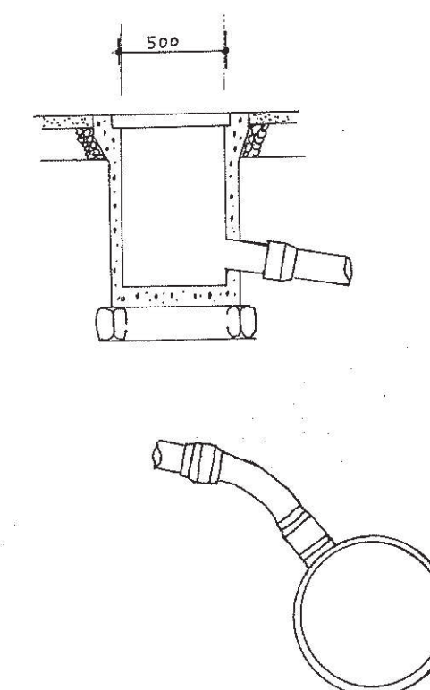
下水本管接續構造図 S:1/30
