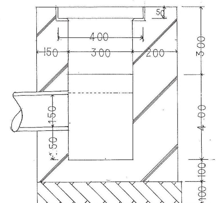
側溝会所構造図 5\frac{1}{10}
