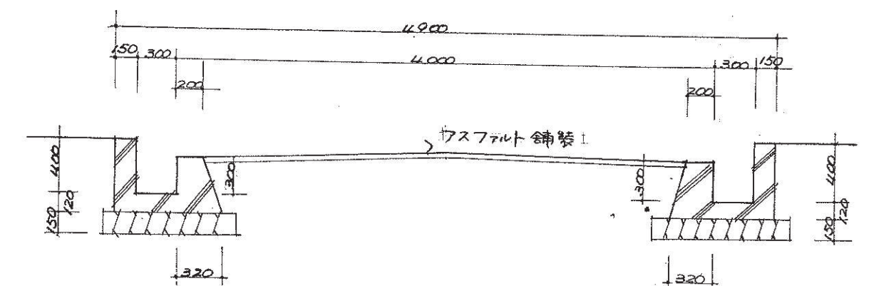
断面図 S = 1/40
