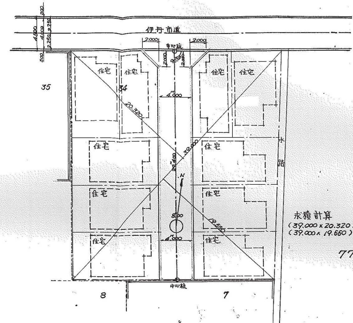
道路平面図 1:300
