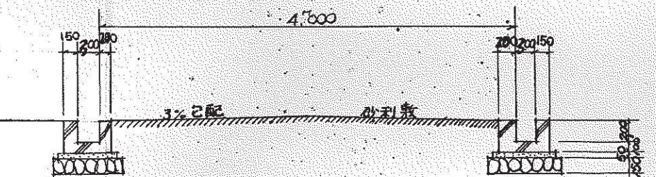
道路横断面図 1:50
