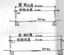
断面図 1:100
