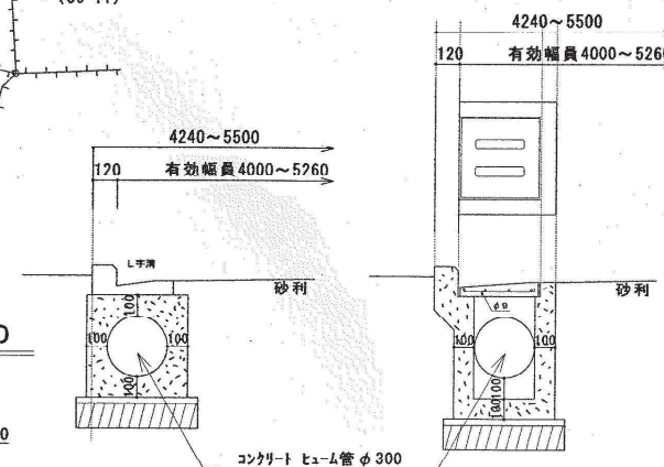
側溝詳細図 S = 1 / 20
