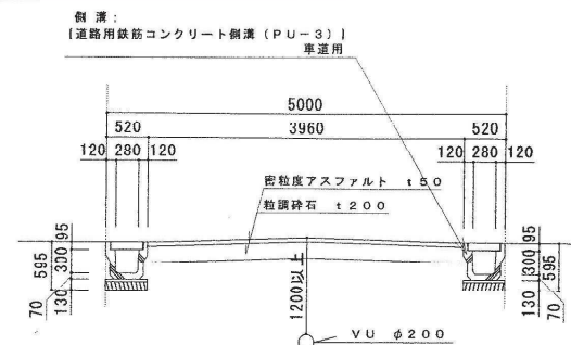
道路標準断面図 S = 1/50
