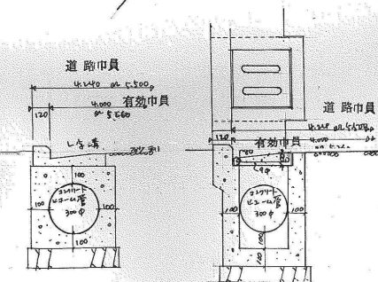
側溝 詳細図 1:20
