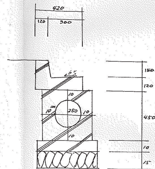
上-△管断面图 5:20
