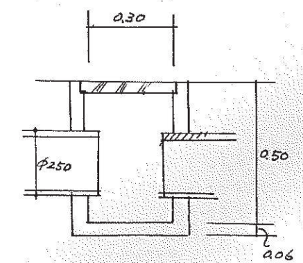
会所断面 S1:20
