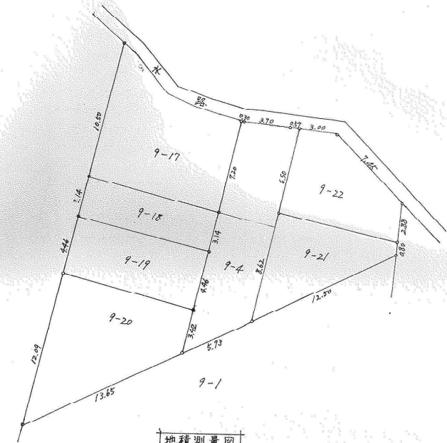
地積測量図
