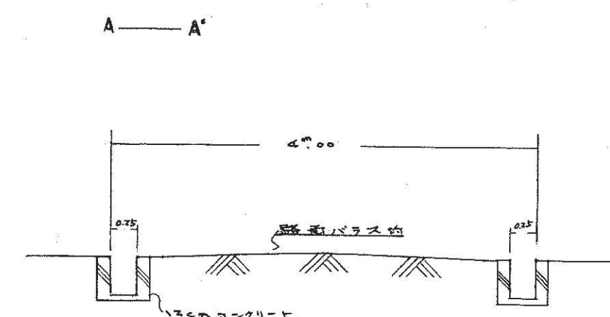
断面図 S=1:50
