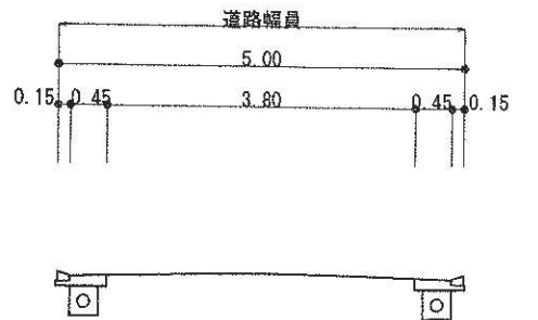
道路横断面図 S=1:100
