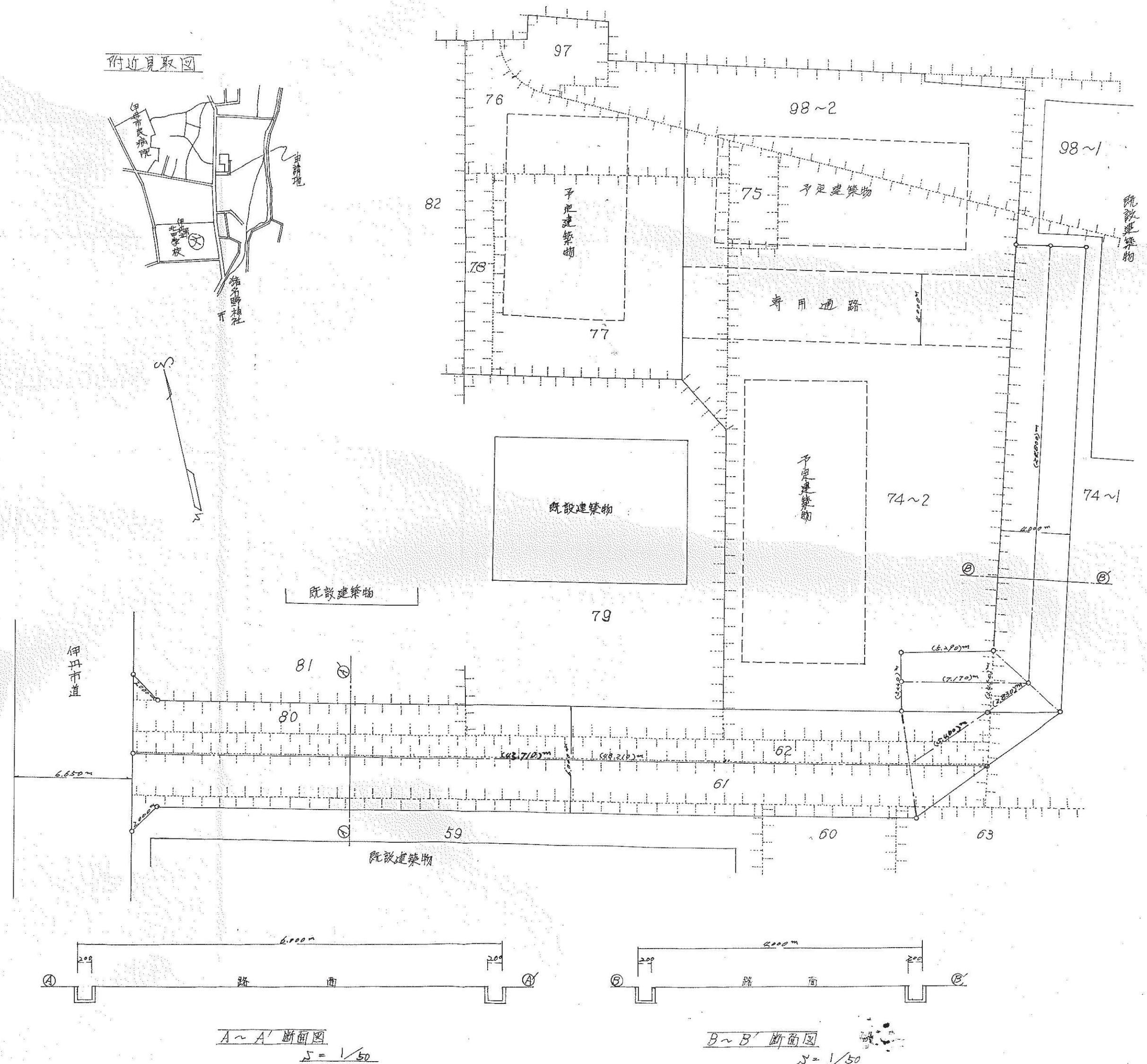
配置図
