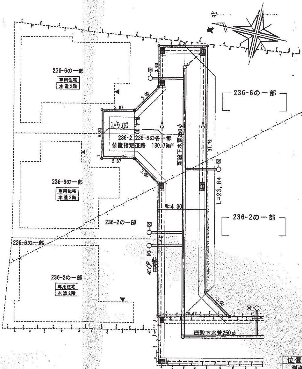
道路計画平面図 S=1/200
