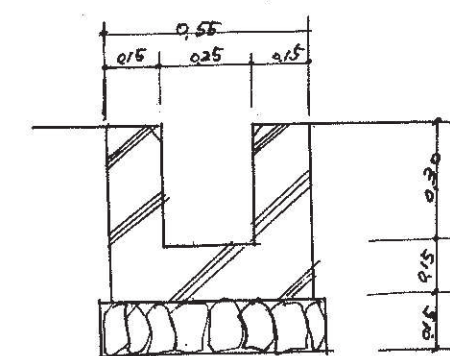
A-A 道路断面 縮尺 1:100
