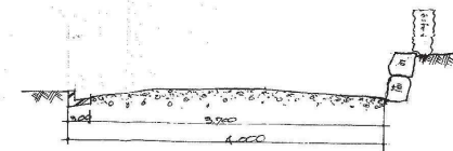
A-A' 断面図 S=1/50
