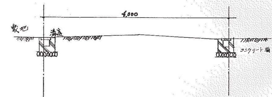
A-B 断面图
