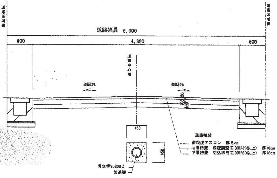
位置指定道路横断面図 S=1/50
