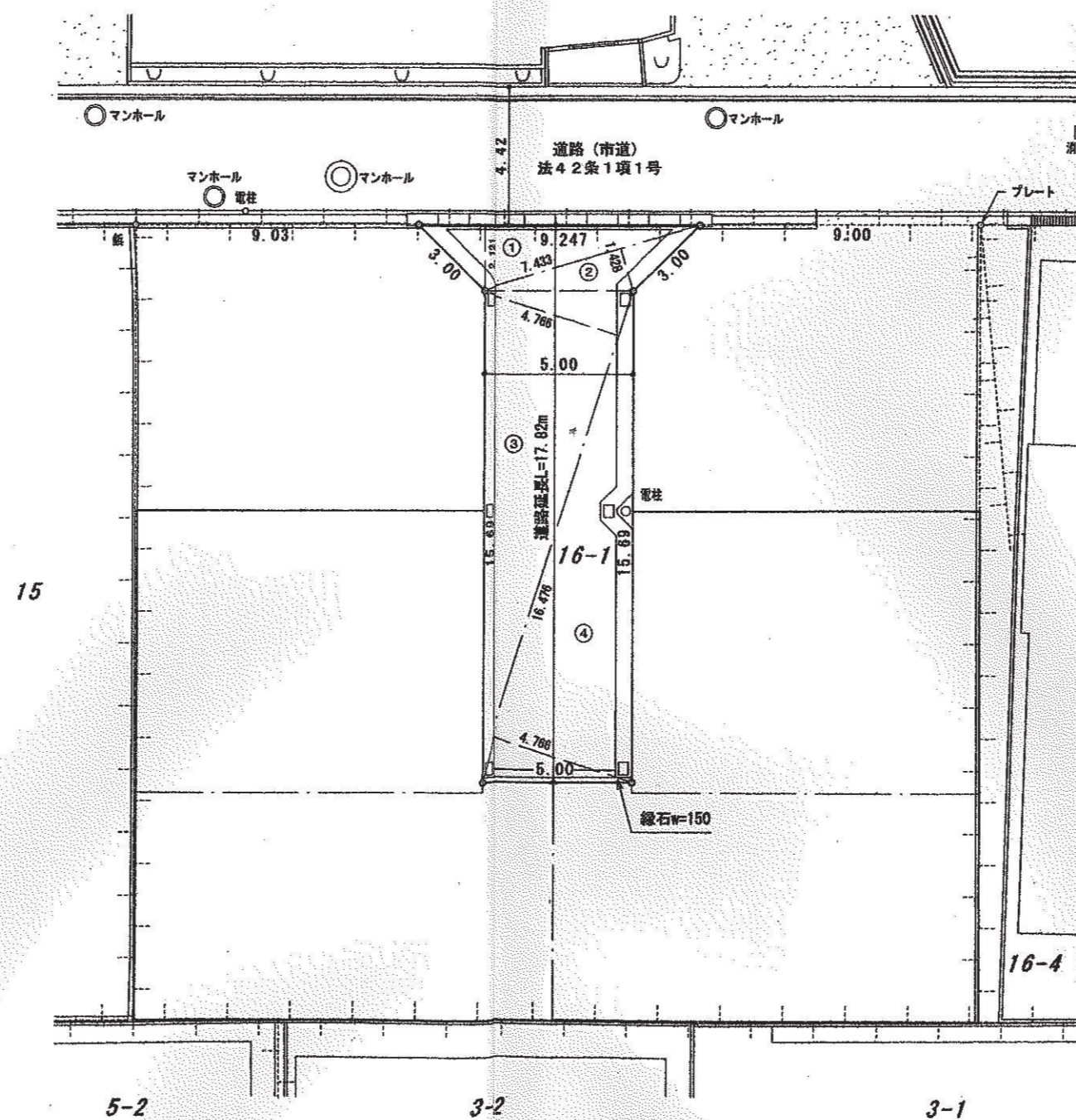
平面図 S=1/200
