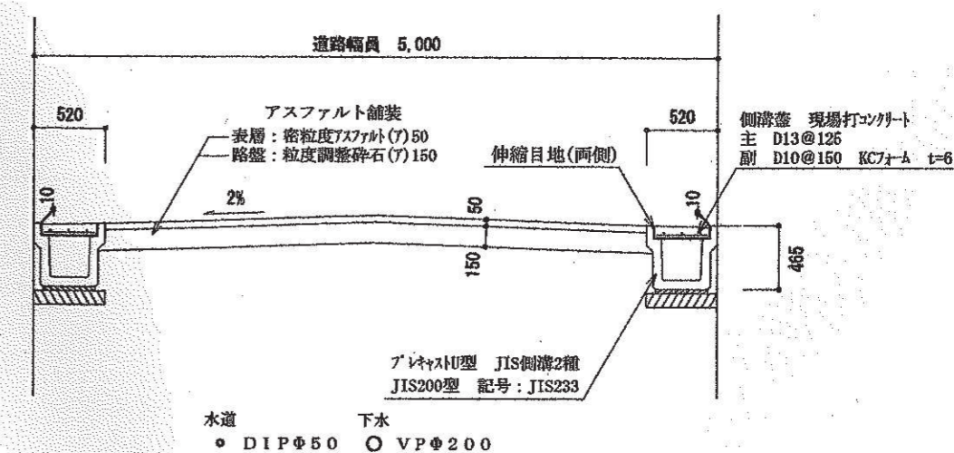
位置指定道路構造図
