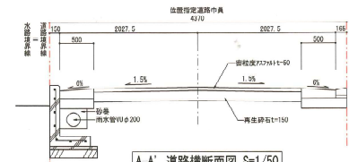
A-A' 道路横断面図 S=1/50
