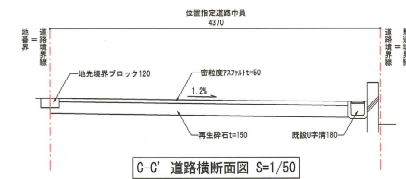
C-C' 道路横断面図 S=1/50
