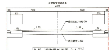
B-B' 道路横断面図 S=1/50
