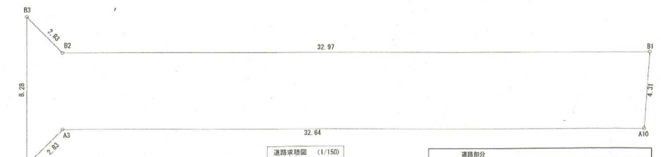
道路求積図 (1/150)
