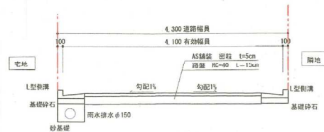
道路標準断面図 (1/50)
