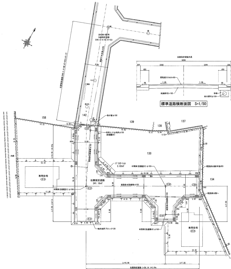
道路平面図 S=1/500
