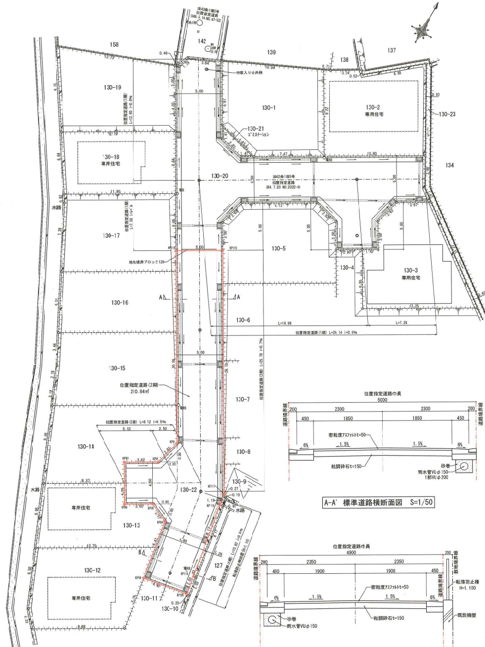
道路平面図 S=1/200
