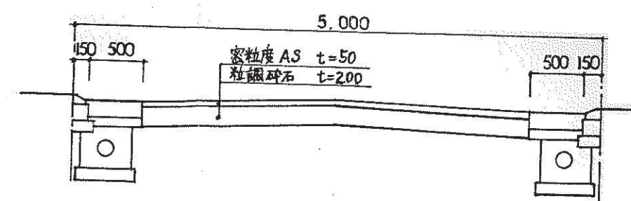
標準断面図 SC = 1/50
