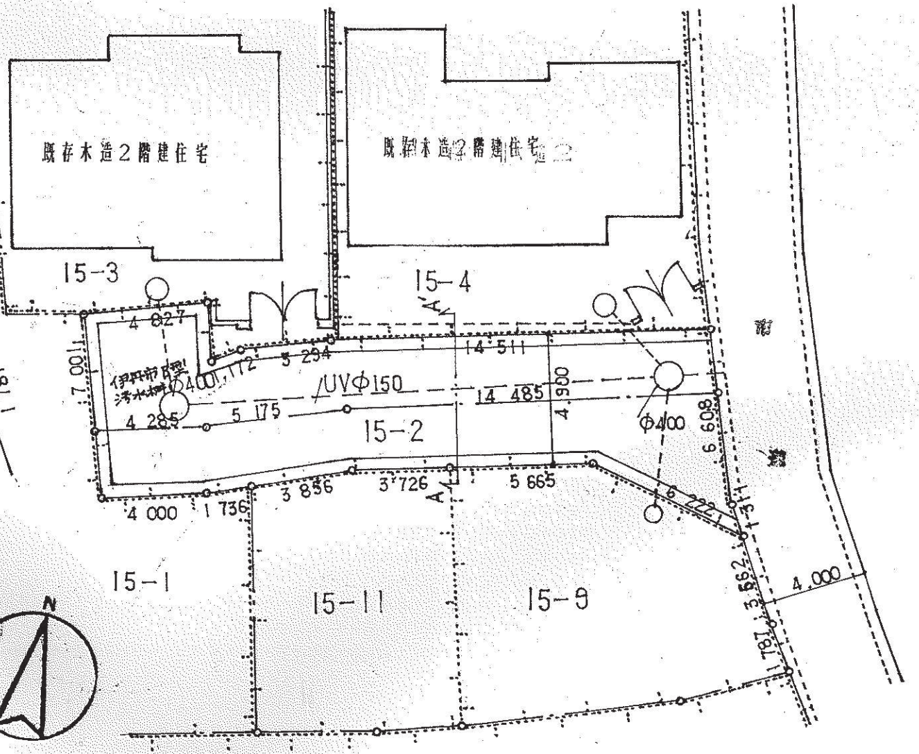
平 面 圖 S=1/200
