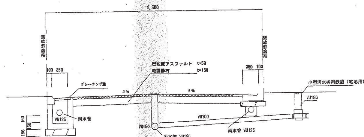
横断道路排水図 S=1/50
