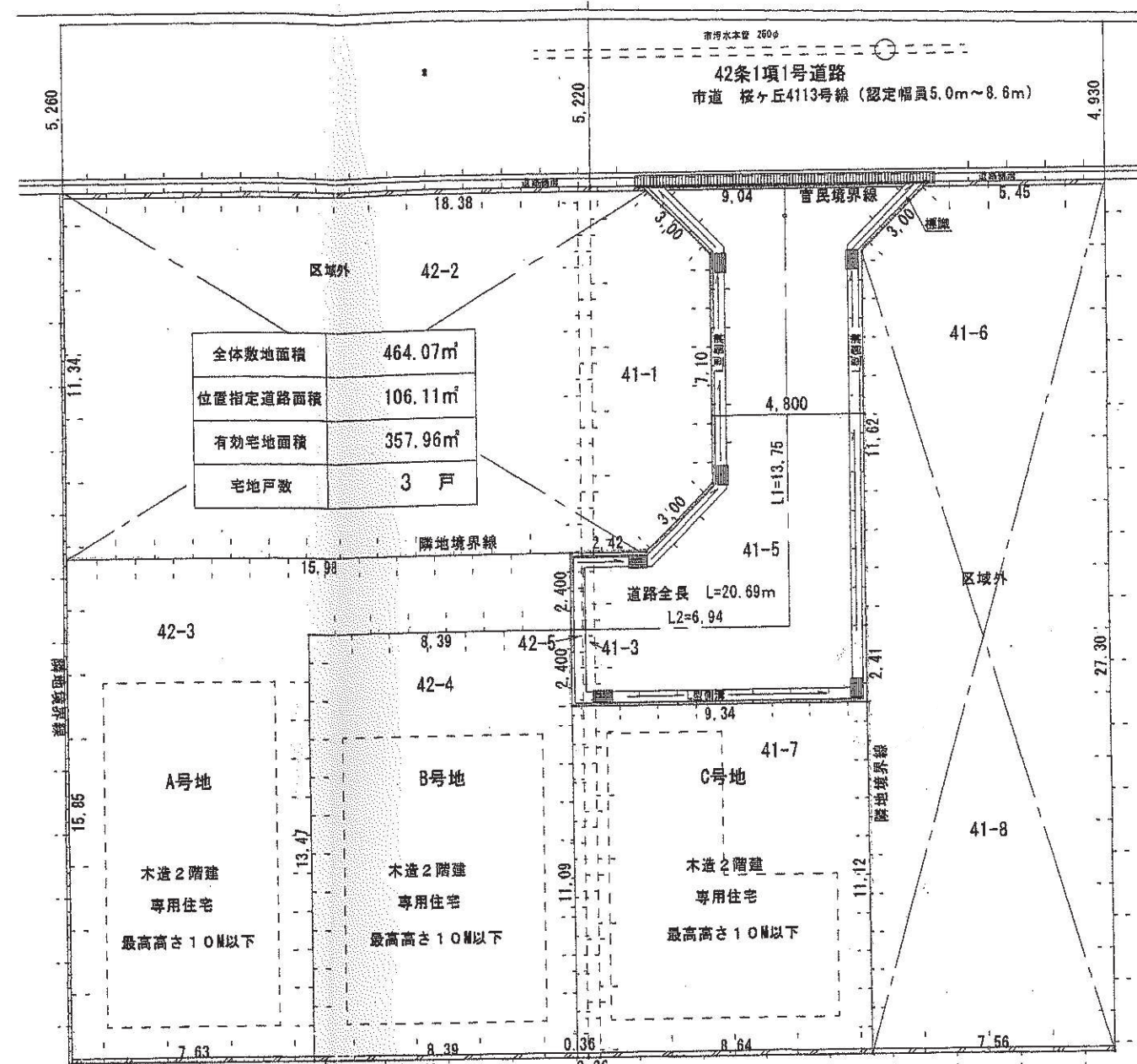
道路平面図 S:1/200
