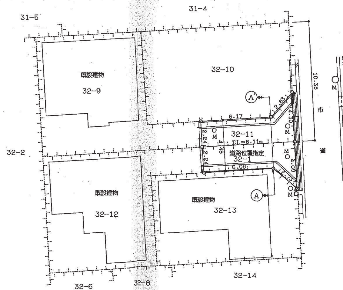
平面図 S = 1 : 200
