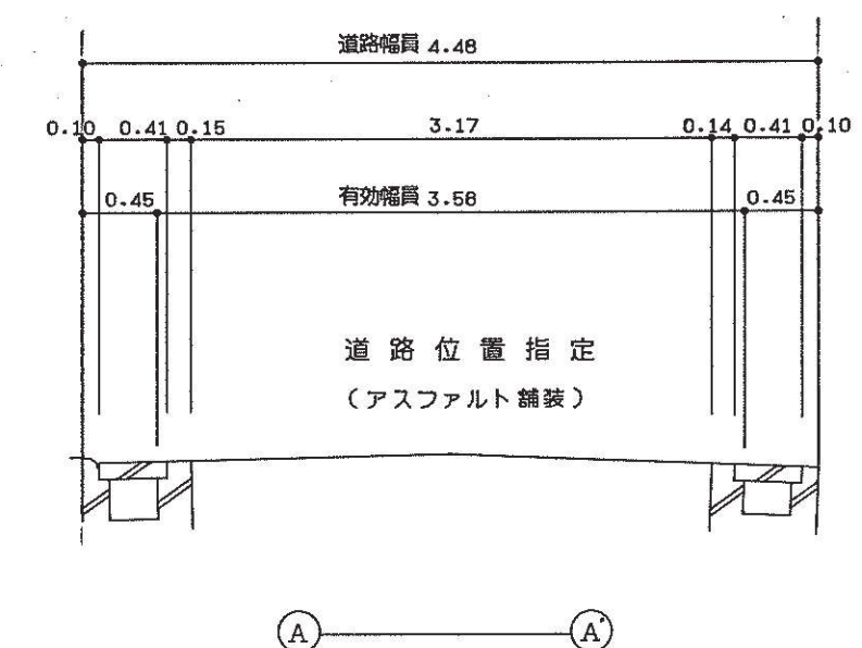
断面図 S = 1 : 50
