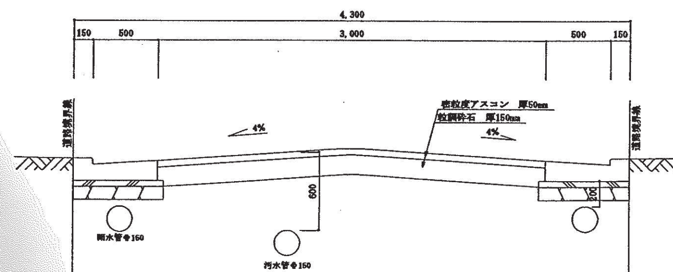
道路断面詳細図 S=1 : 30
