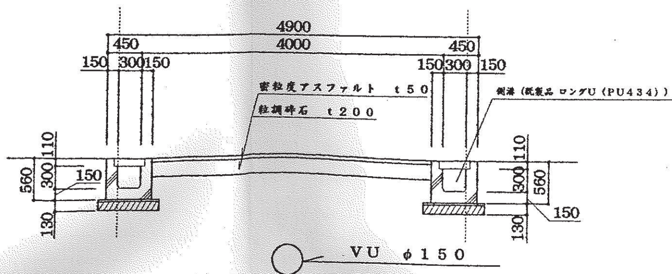
道路標準断面図 S=1/50
