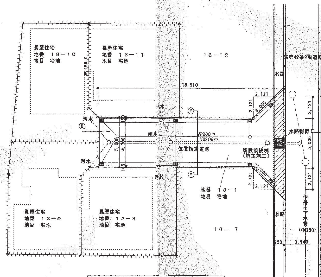
道 路 平 面 図 S=1/200
