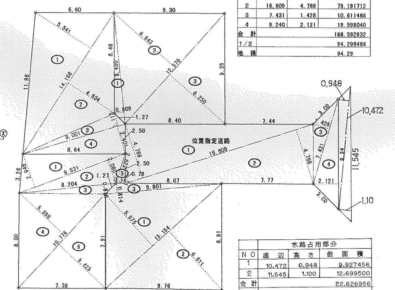
敷 地 求 積 図 S=1/200
