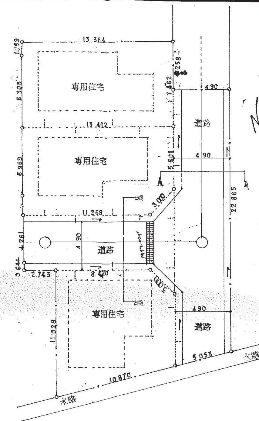
平 面 図 S=1/200
