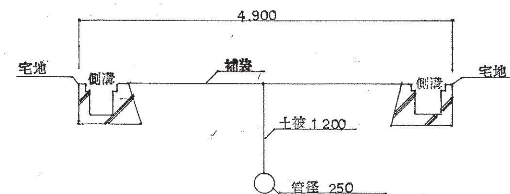
A—A B—B 断面図 1:500
