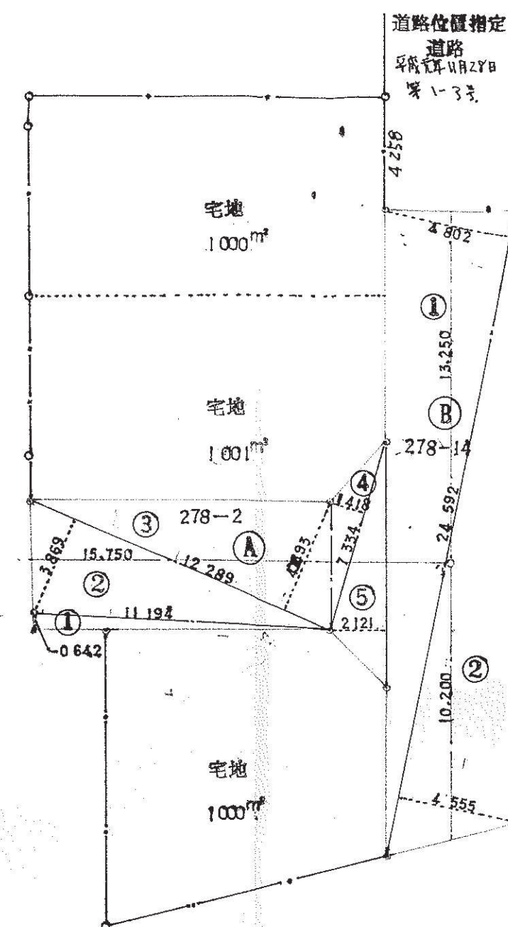
実 測 図 S=1/200
