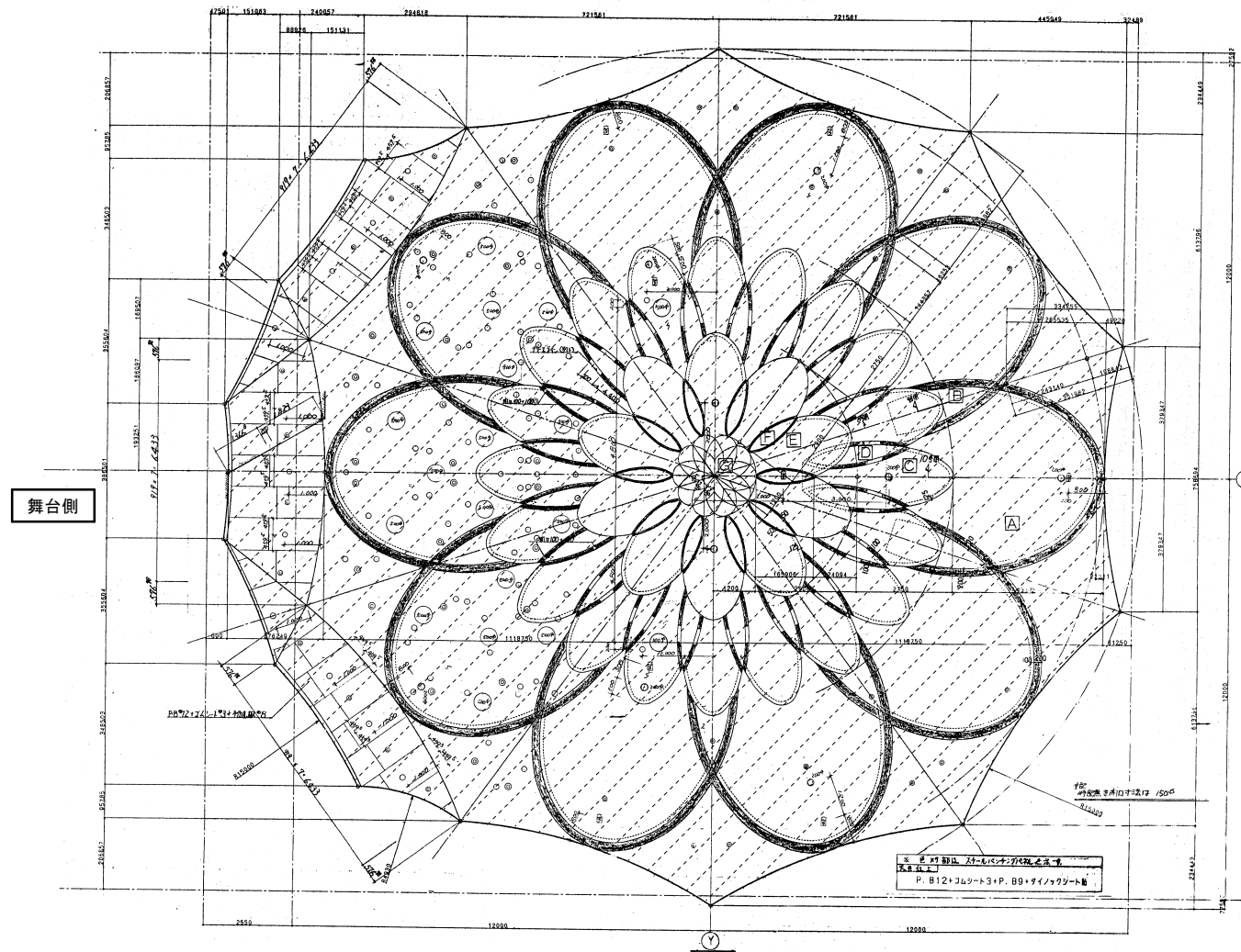
大ホール天井伏図
