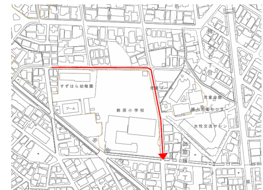
鈴原町地区雨水管渠整備箇所図
