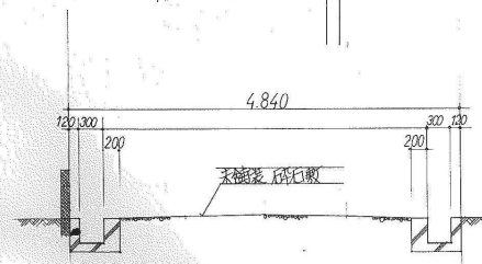
断面図 S-1/50
