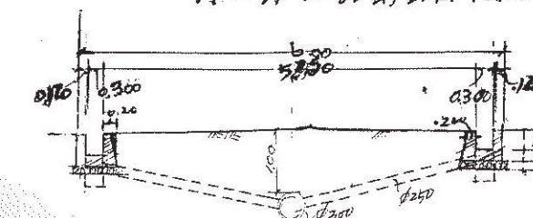
B-B 道路断面図 1:100
