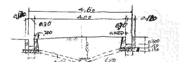
A-A 道路断面図 1:100
