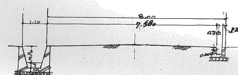
C-C 道路断面図
