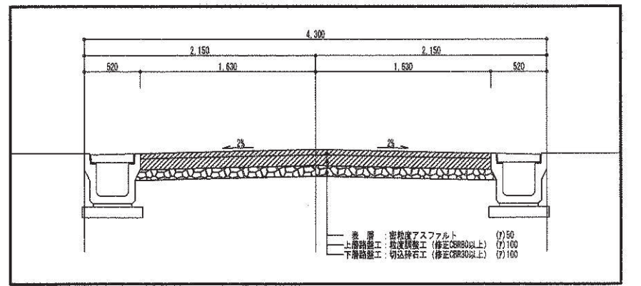
道路標準断面図 S:1/50
