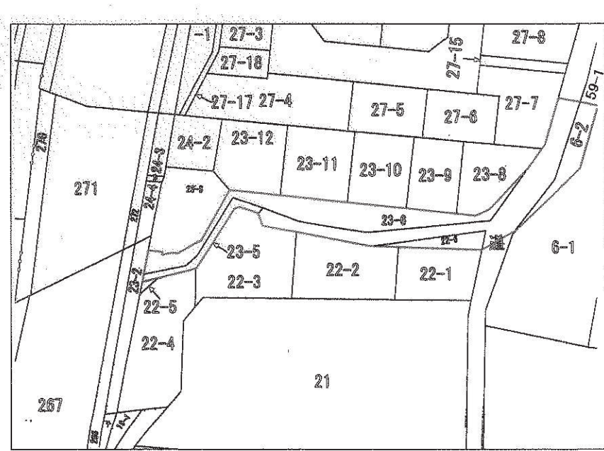
字 限 図 法務局備付け原図からの写し 平成29年12月25日
