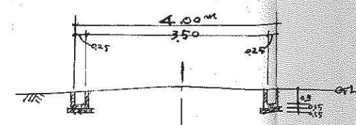
A-A 道路断面 1:100.0m
