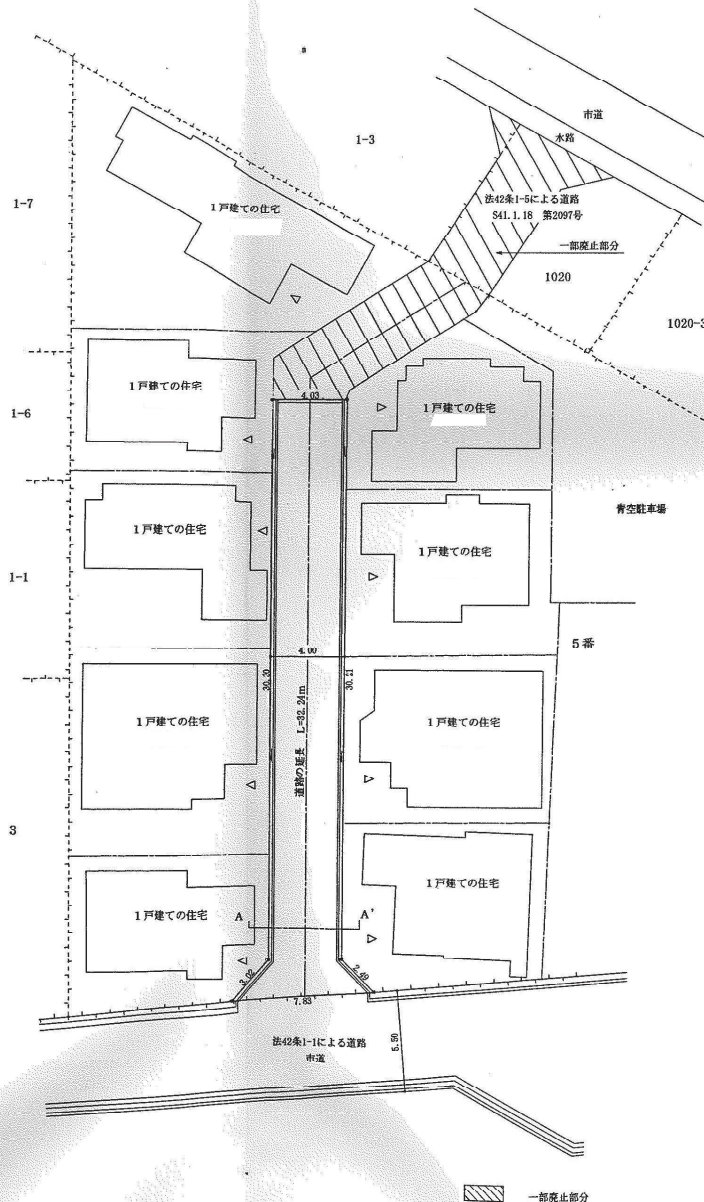
平面図 S:1/200
