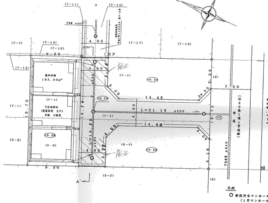
道路平面図 S=1/200
