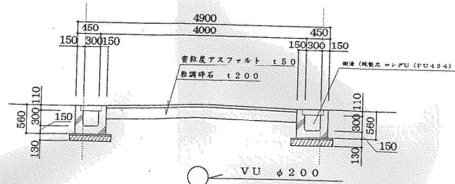
道路標準断面図 S=1/50
