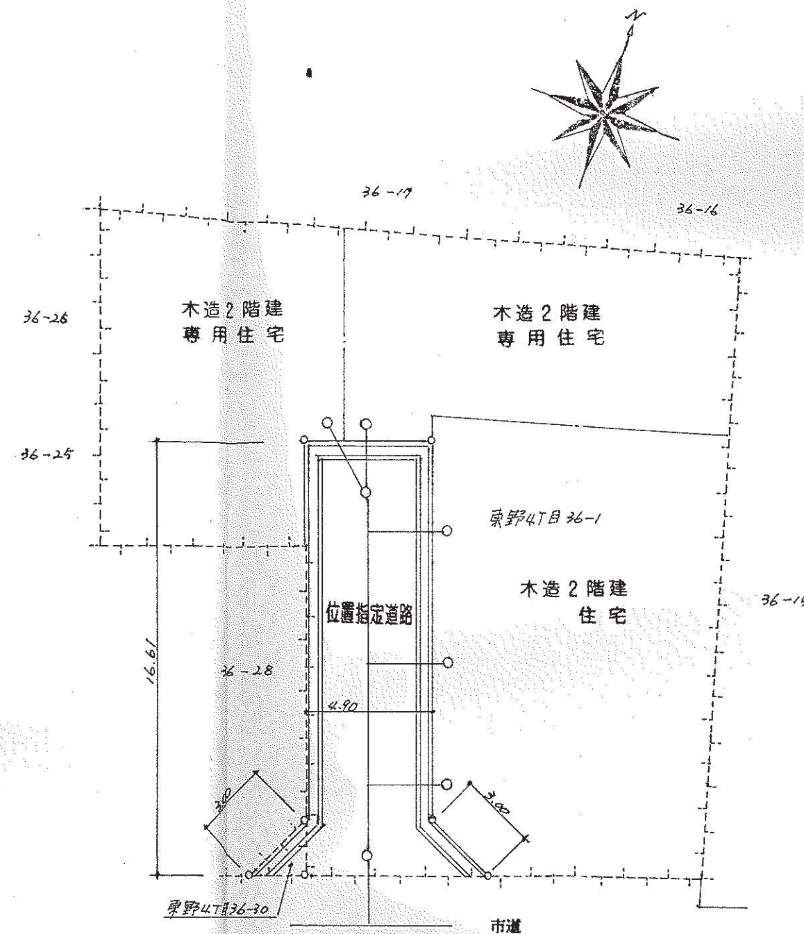
平面図 S=1:200
