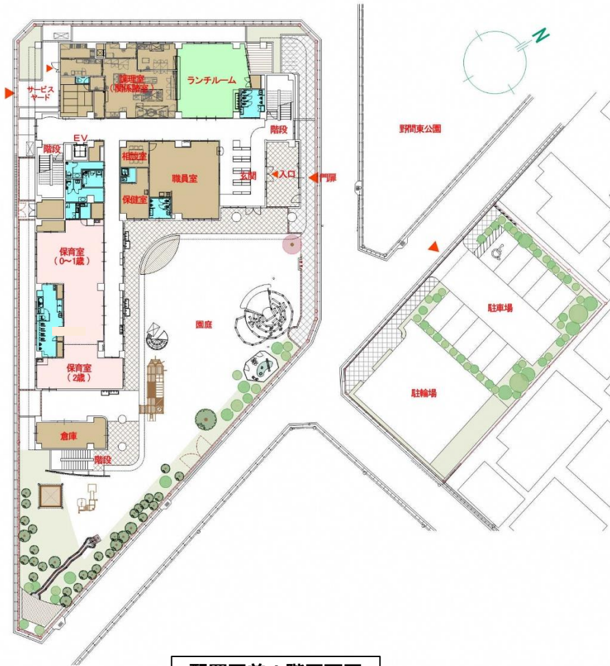
配置図兼1階平面図
