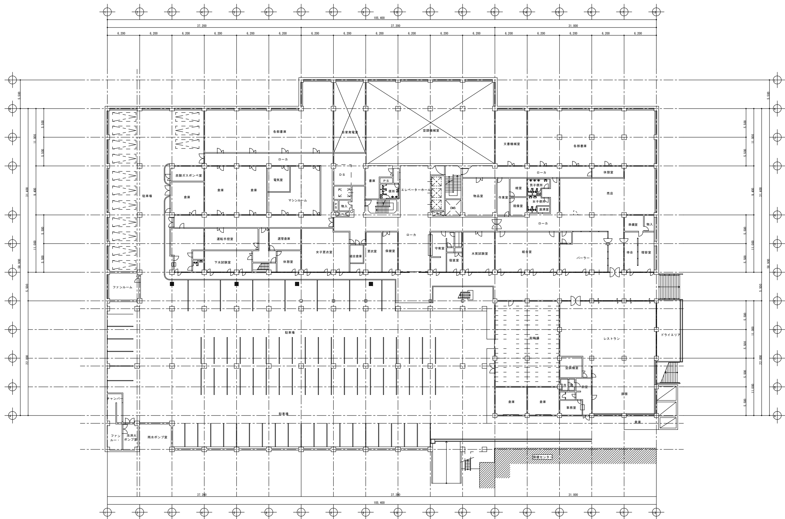
地下1階平面図
