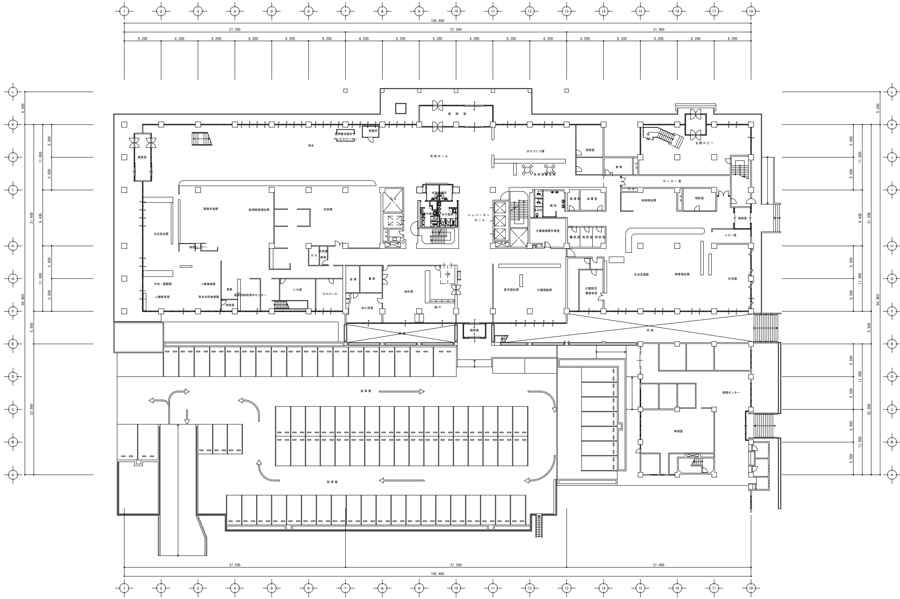
1 階平面図
