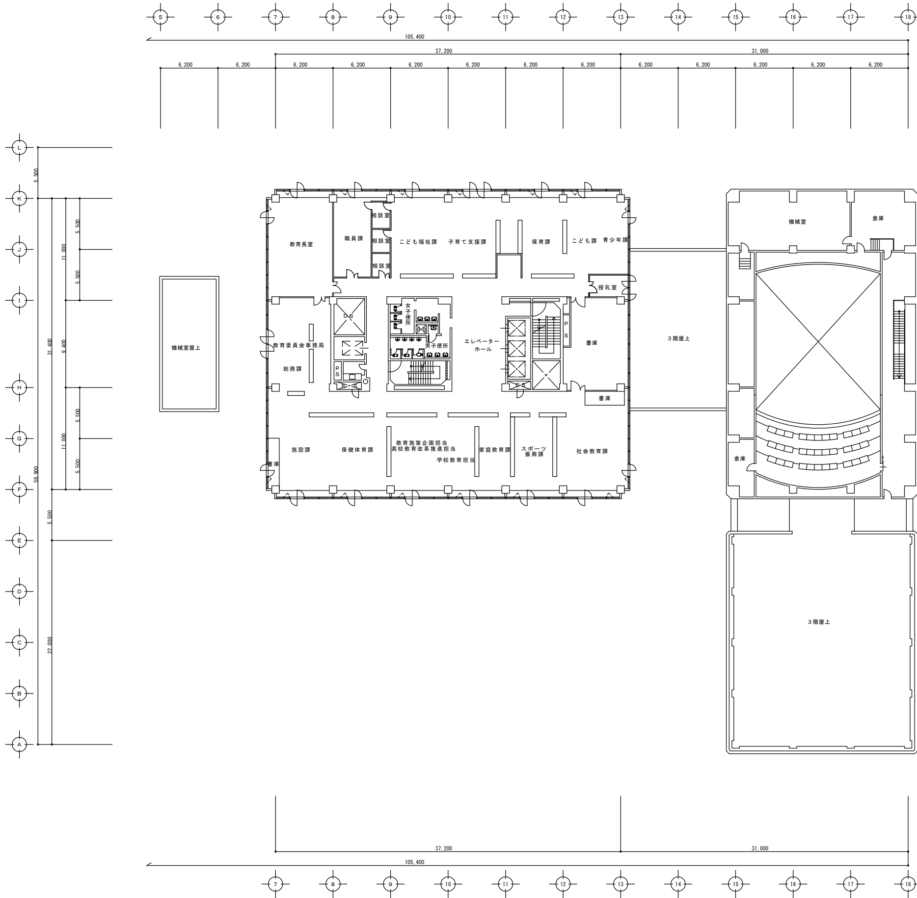
4階平面図
